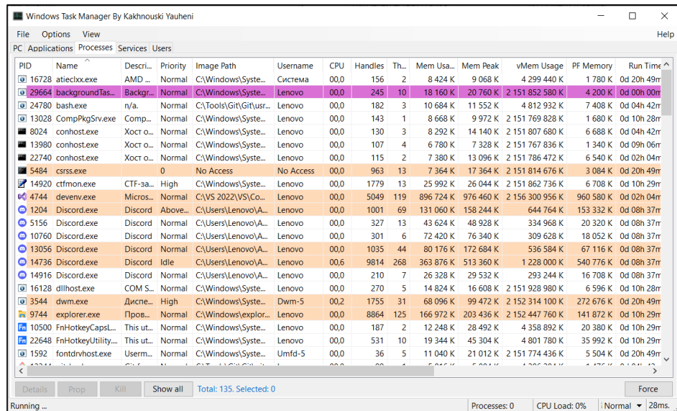
Рисунок 5.12 – Вкладка «Processes»
